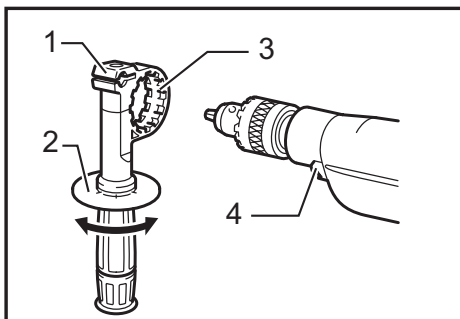
► 1. Base de la empuñadura 2. Empuñadura lateral (mango auxiliar) 3. Dientes 4. Protuberancias
