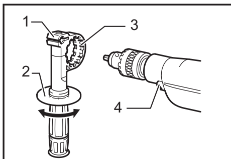
► 1. Base de la poignée 2. Poignée latérale (poignée auxiliaire) 3. Dents 4. Saillies
